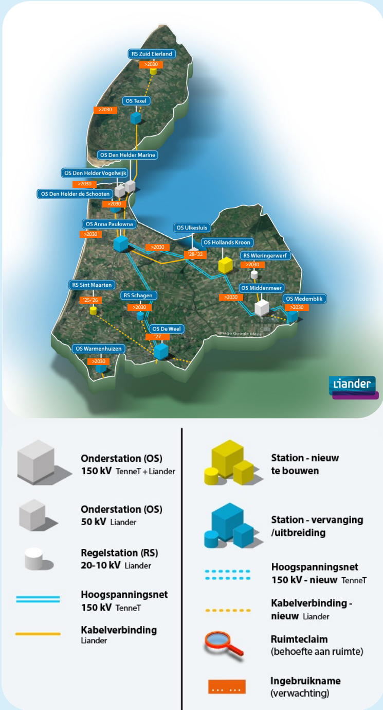
Netsituatie Kop van Noord-Holland (>2MW, huidig en voorzien)
