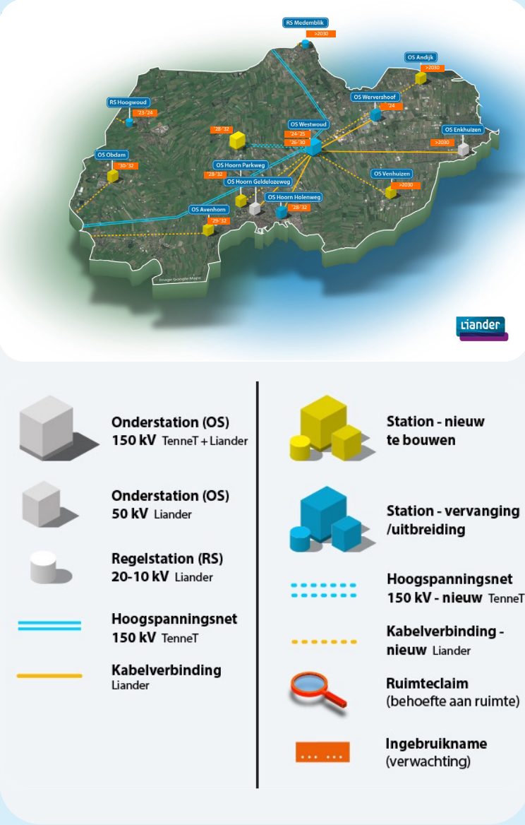
Netsituatie Westfriesland (>2MW, huidig en voorzien)
