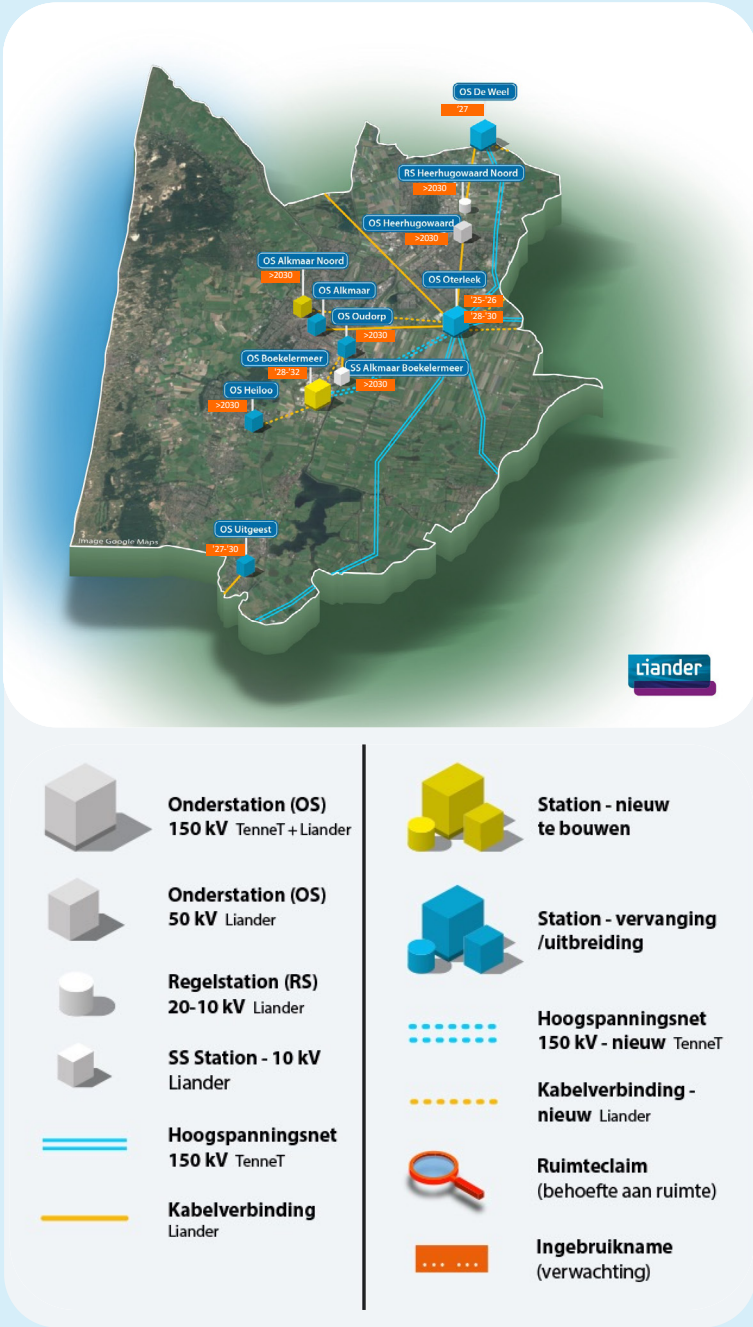
Netsituatie regio Alkmaar (>2MW, huidig en voorzien)
